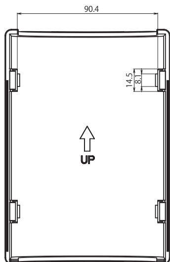
詳細図 A
