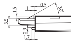
詳細図 B
