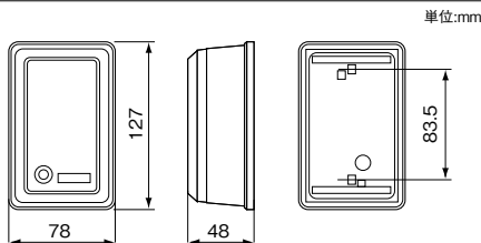
外形寸法図
