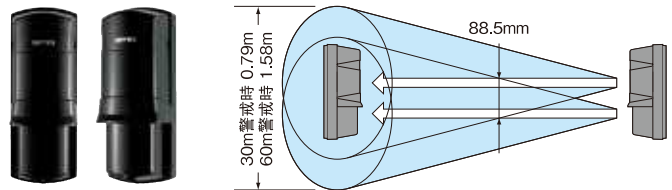
外形寸法図
