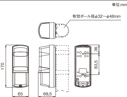
外形寸法図
