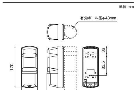
外形寸法図
