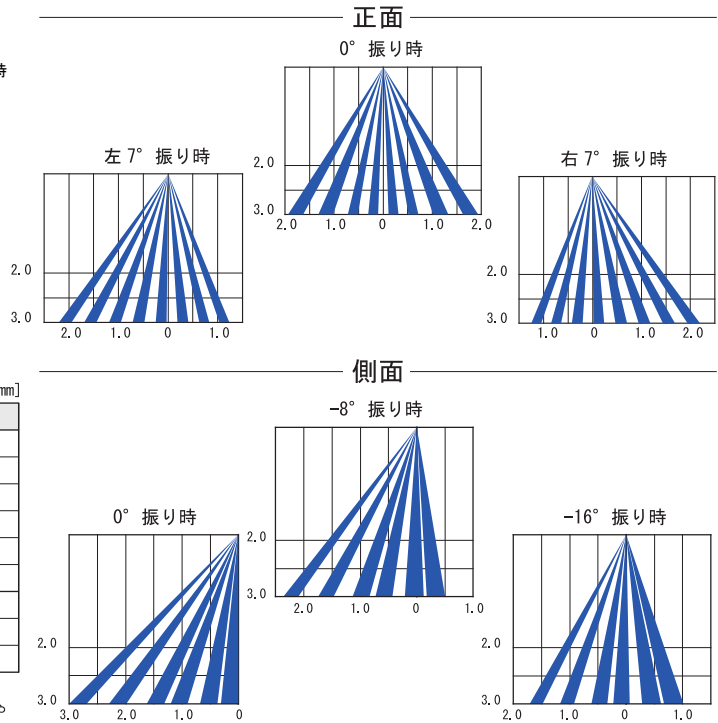
検出エリア（補助エリア）（単位：m）
