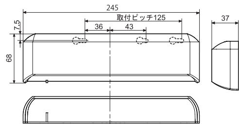
防雨カバー(L)
