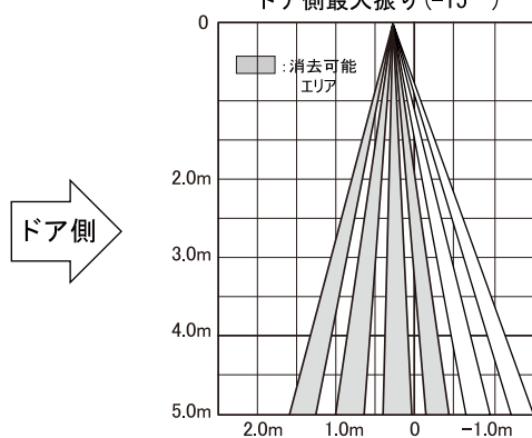
ドア側最大振り(-15°)
