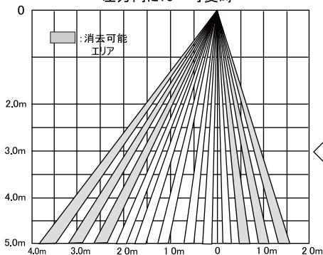
左方向に10° 可変時
