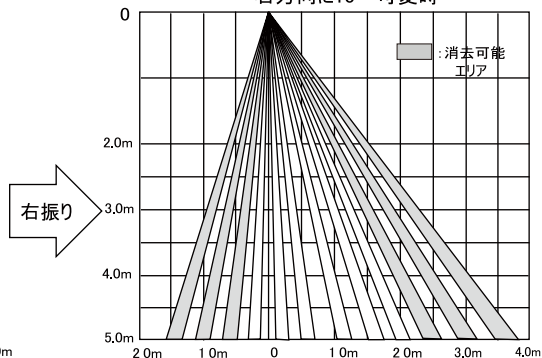
右方向に10° 可変時
