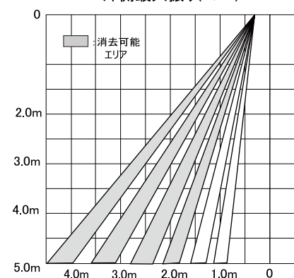
外側最大振り(10°)
