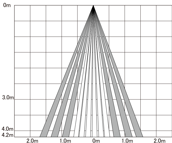
正面図
