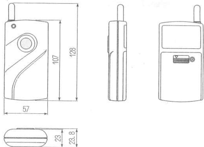
外形寸法図
