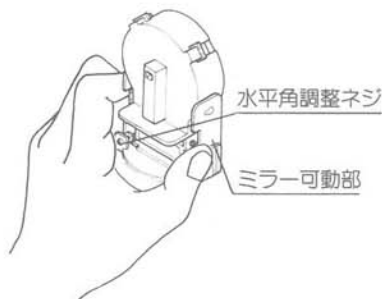
(水平角調整)
