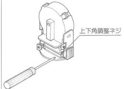
(上下角調整)
