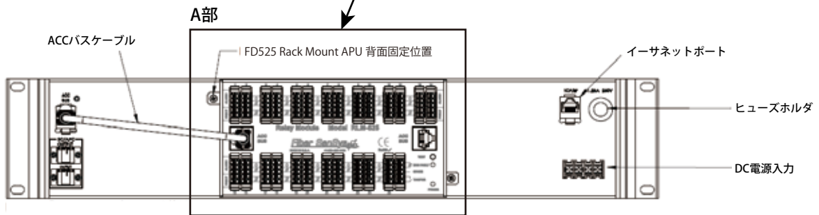
FD525 Rack Mount APU 背面へのリレーモジュールユニット装着図
